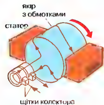
Електрогенератор Робота генератора постійного струму
